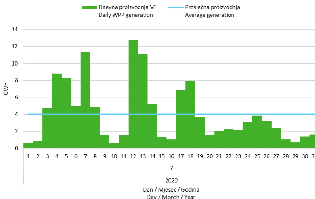
Slika 5 Dnevna proizvodnja svih vjetroelektrana u srpnju 2020. godine
