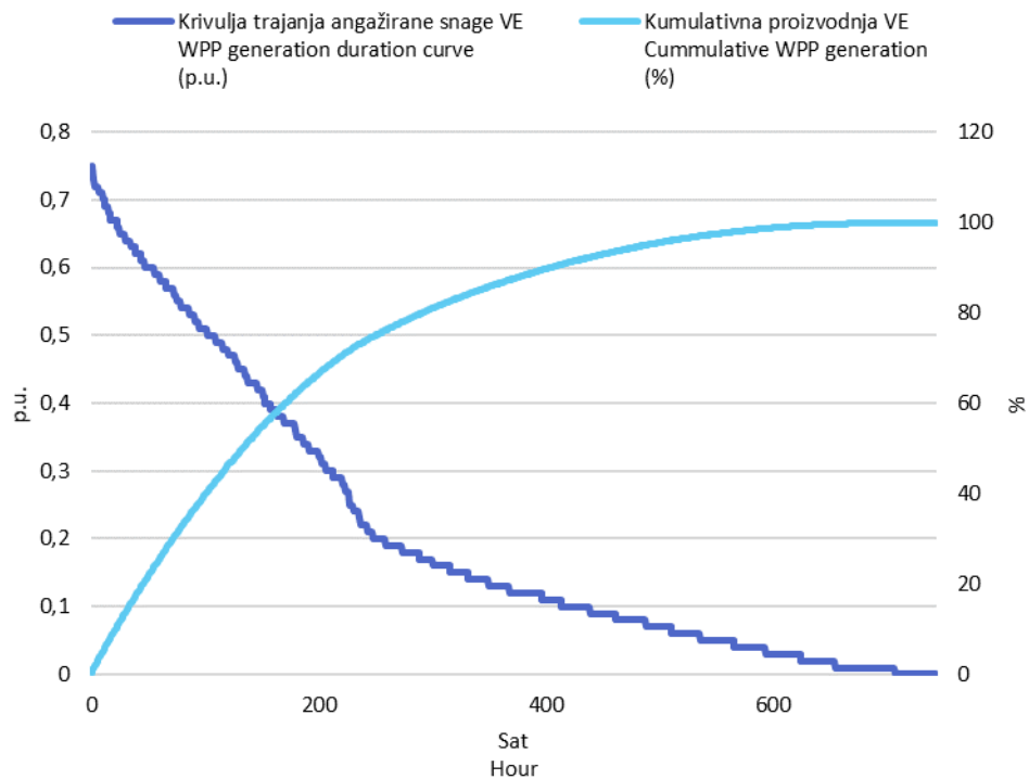
Slika 3 Krivulja trajanja angažirane snage svih VE i kumulativna proizvodnja VE u srpnju 2020. godine u jediničnim vrijednostima
