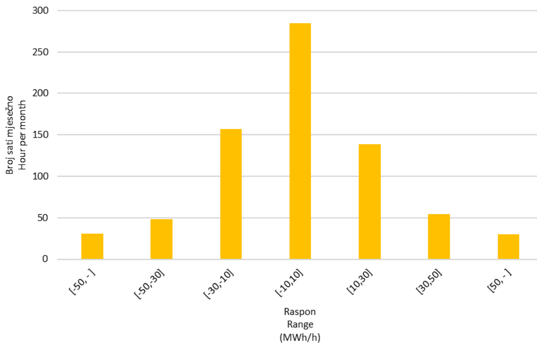
Slika 10 Statistička raspodjela satnih promjena proizvodnje VE u srpnju 2020. godine
