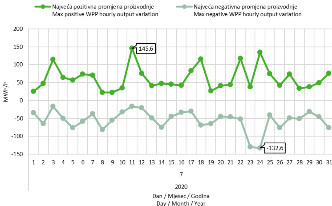
Slika 9 Maksimalna pozitivna i maksimalna negativna promjena satne proizvodnje VE u srpnju 2020. godine
