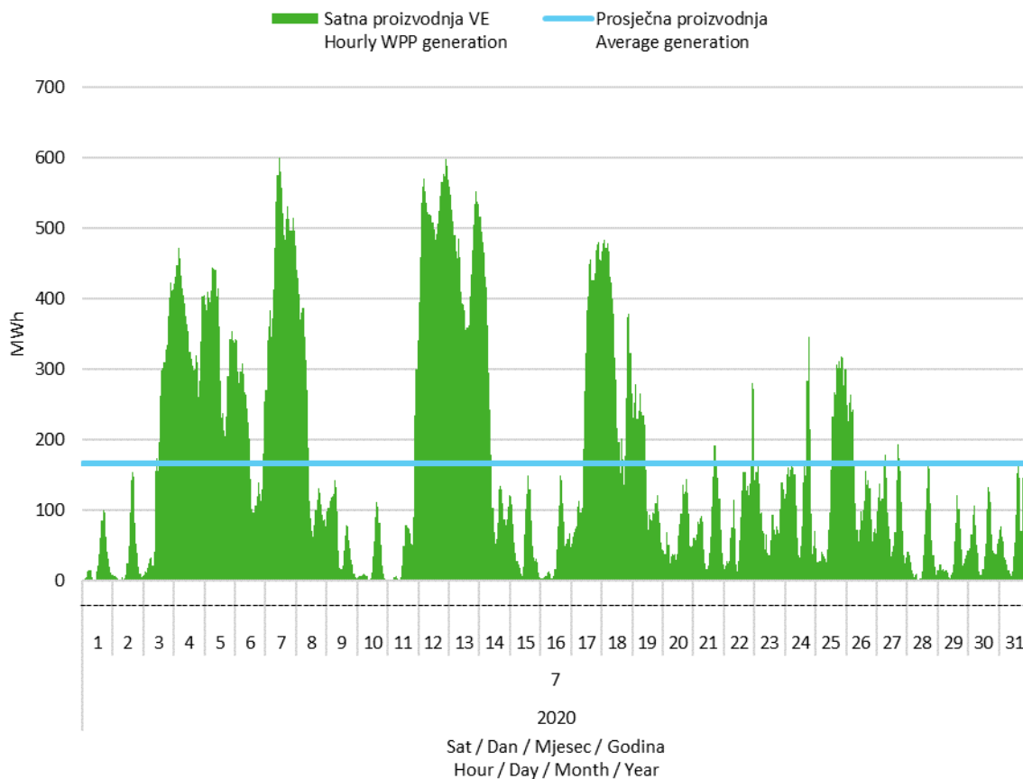
Slika 2 Satna proizvodnja svih vjetroelektrana u srpnju 2020. godine
