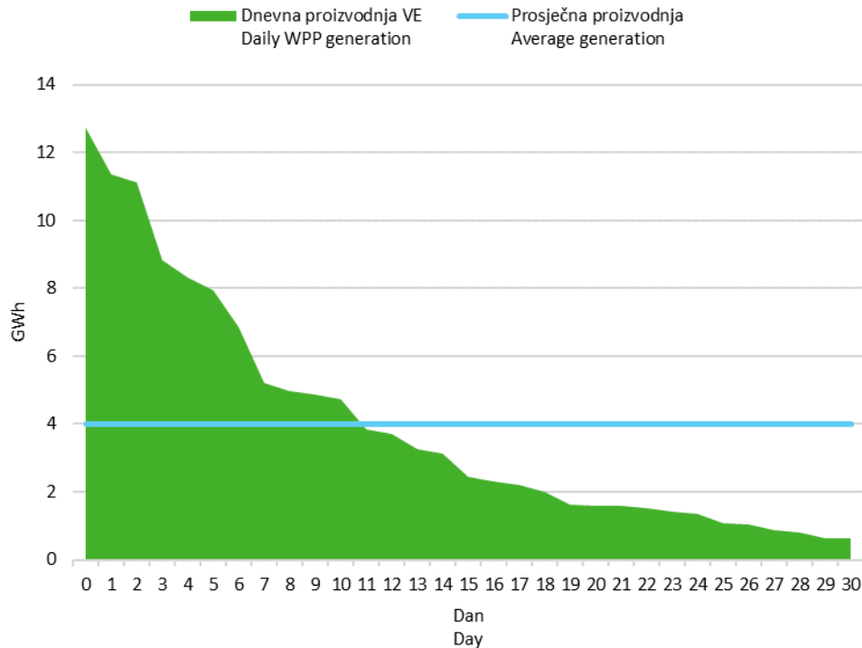
Slika 6 Krivulja trajanja dnevne proizvodnje vjetroelektrana u srpnju 2020. godine
