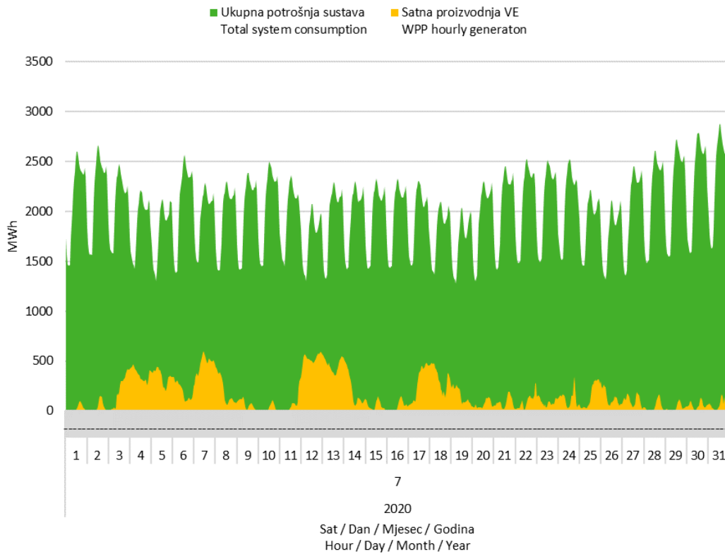
Slika 7 Usporedba satnog dijagrama opterećenja sustava i proizvodnje vjetroelektrana u srpnju 2020. godine
