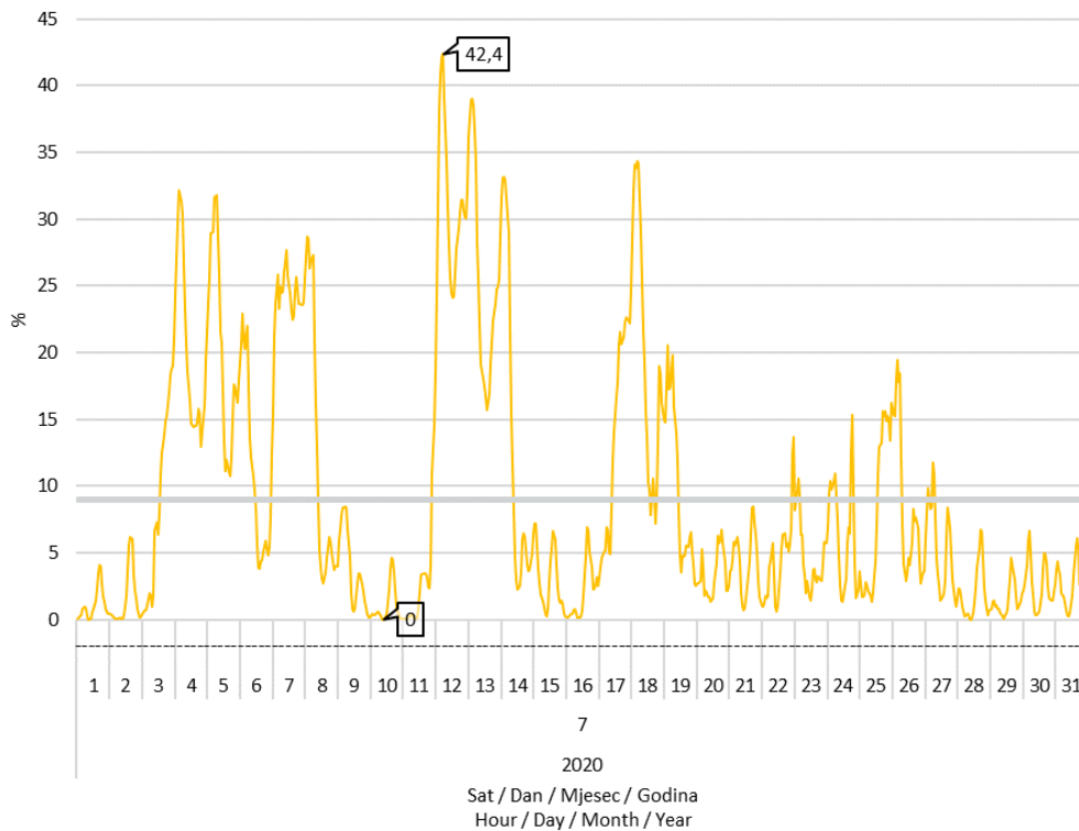
Slika 8 Udio proizvodnje vjetroelektrana u pokrivanju satnog opterećenja elektroenergetskog sustava u srpnju 2020. godine
